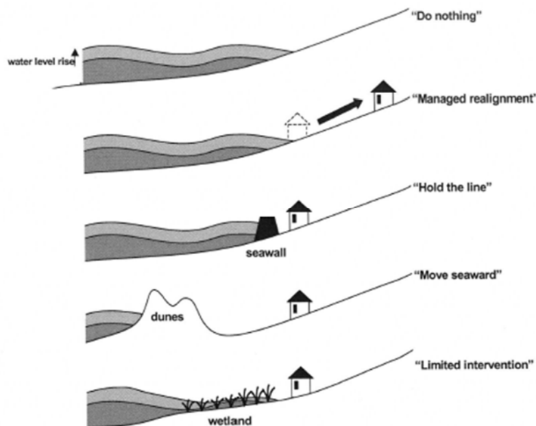
Modos de actuación frente al nivel del mar en la costa. Fuente: IPCC
